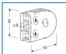
Glasklemme H 40,0 x B 50,0 x T 24,0 mm Anschluss gerade
