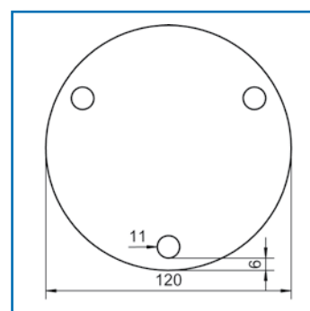
V2A Ronden mit Lochungen, einseitig 240 Korn geschliffen. Einzeln im Polybeutel verpackt. 120,0 x 8,0
