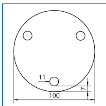
V2A Ronden mit Lochungen, einseitig 240 Korn geschliffen. Einzeln im Polybeutel verpackt. 100,0 x 8,0
