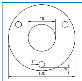
V2A Ronden mit Lochungen, einseitig 240 Korn geschliffen. Einzeln im Polybeutel verpackt. 120,0 x 6,0
