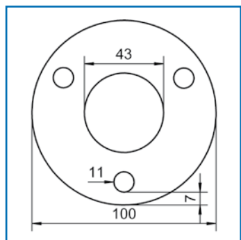
V2A Ronden mit Lochungen, einseitig 240 Korn geschliffen. Einzeln im Polybeutel verpackt. 100,0 x 6,0
