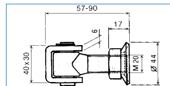
Torband zum Anschweißen Maße und Preise siehe nebenstehende Tabelle
