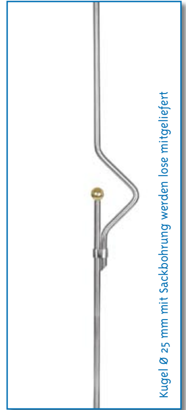
Kugel: Messing Art.-Nr. 1865 Kugel: VA Art.-Nr. 1875
